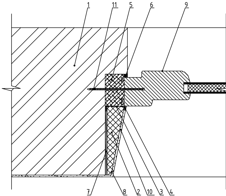
Вузол докового примикання дверної конструкції до стіни без утеплення
