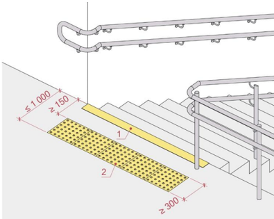
Схема влаштування тактильних елементів
