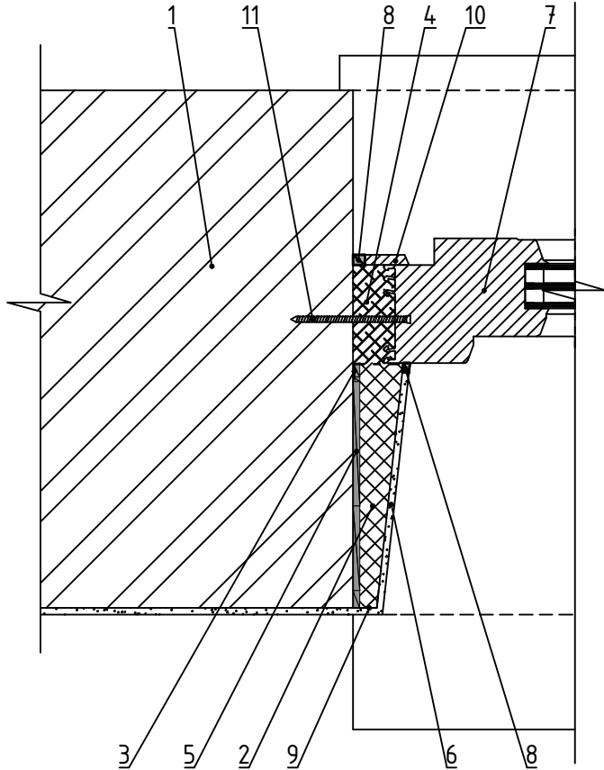
Вузол докового примикання віконної конструкції до не утепленої стіни без четверті
