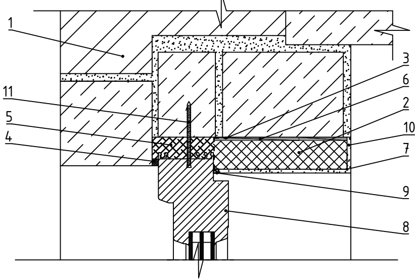
Вузол примикання віконної конструкції до не утепленої стіни без четверті в зоні перемички
