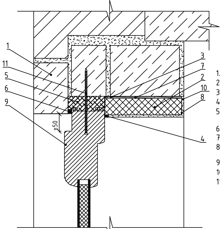
Вузол примикання віконної конструкції до не утепленої стіни без четверті
