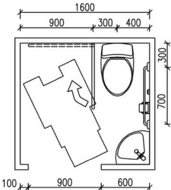
Схема влаштування санітарного вузла
