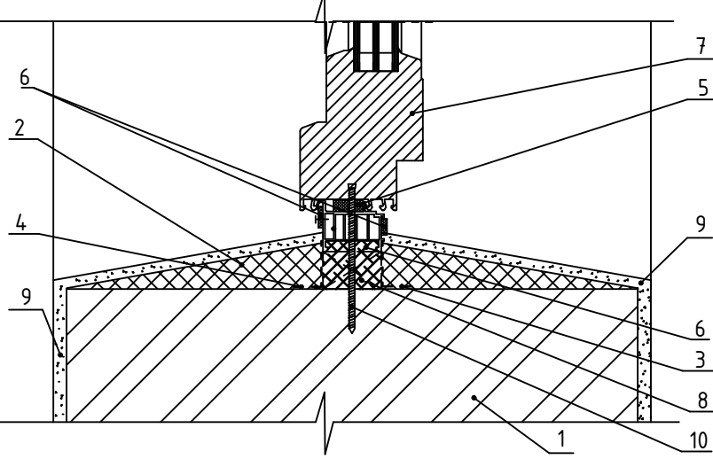
Вузол примикання віконної конструкції до не утепленої стіни без четверті
